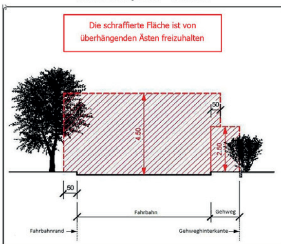
Lichtraumprofil – Strasse
